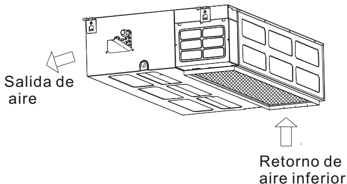
1. Retorno de aire inferior
