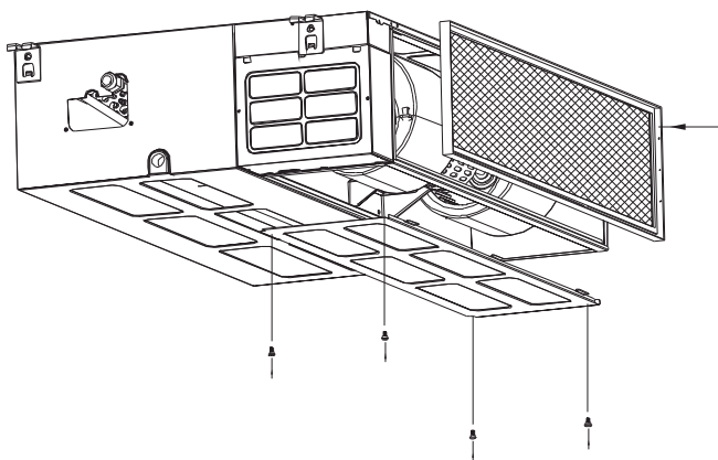
3. Coloque la tapa posterior en la parte inferior de la unidad, donde estaban colocados los filtros
