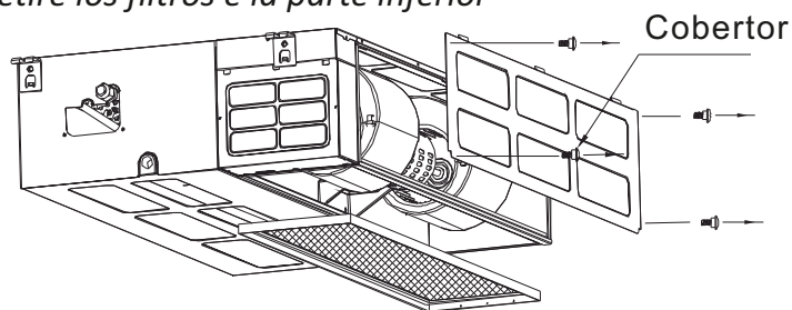
2. Afloje la tuerca y desmonte la tapa posterior. Luego retire los filtros e la parte inferior
